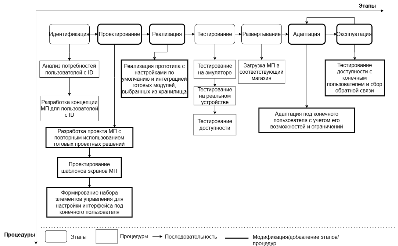
Рисунок 2.1 — Этапы и процедуры ЖЦ МП для людей с ИН
