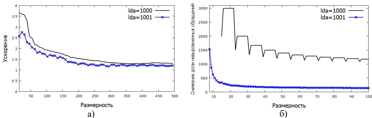
Рисунок 18 – Полученные метрики ПС: ускорение (а), снижение доли невыровненных обращений (б)
