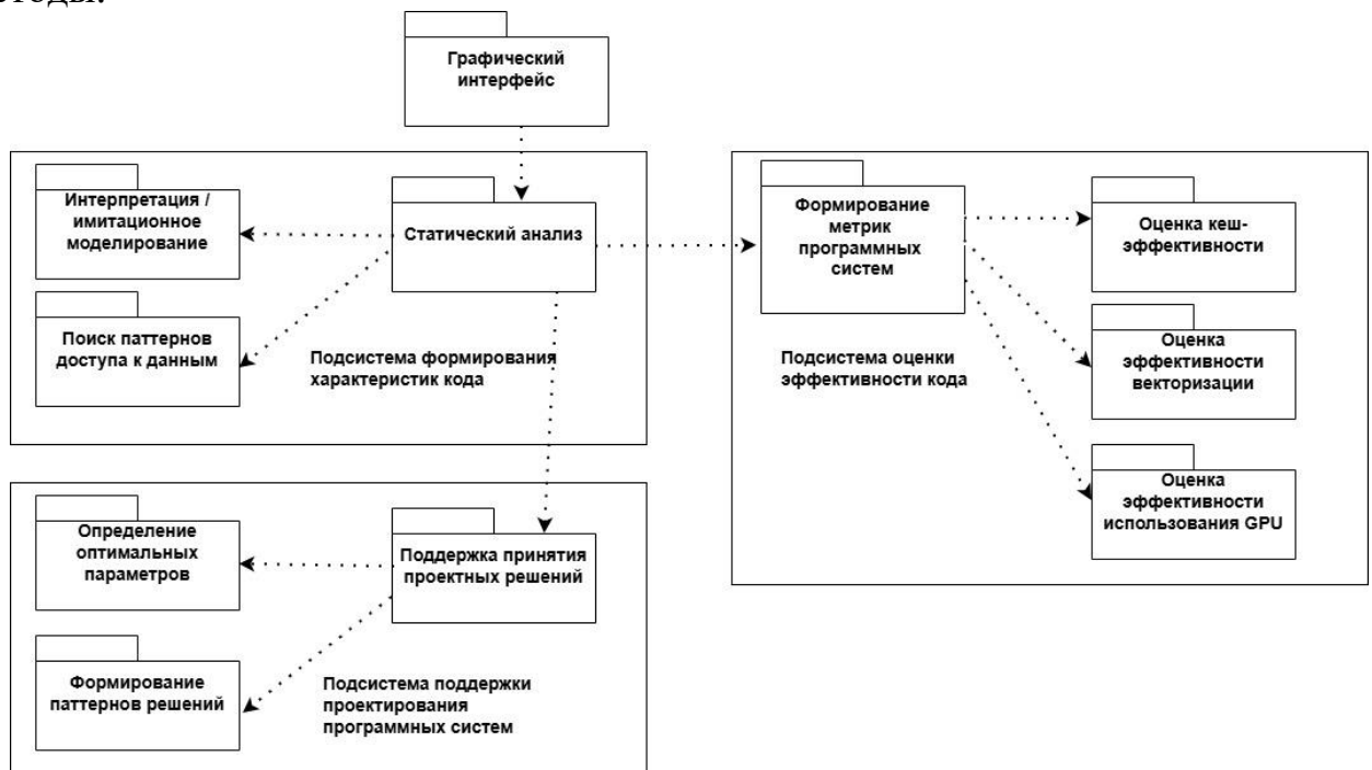
Рисунок 20 - Архитектура системы поддержки ЖЦ проектируемых ПС Система состоит из трех основных подсистем.
