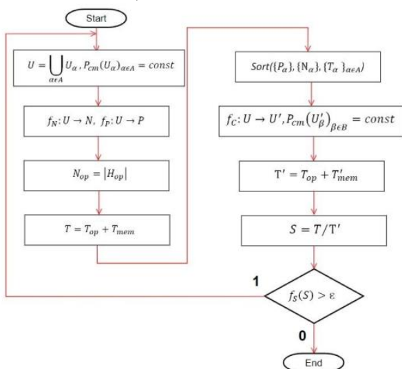
Рисунок 12 - Метод повышения эффективности использования ПП
