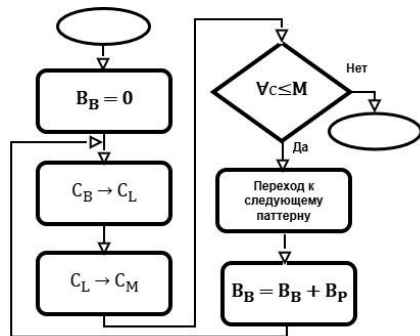
Рисунок 9 – Метод количественной оценки метрик ПС
