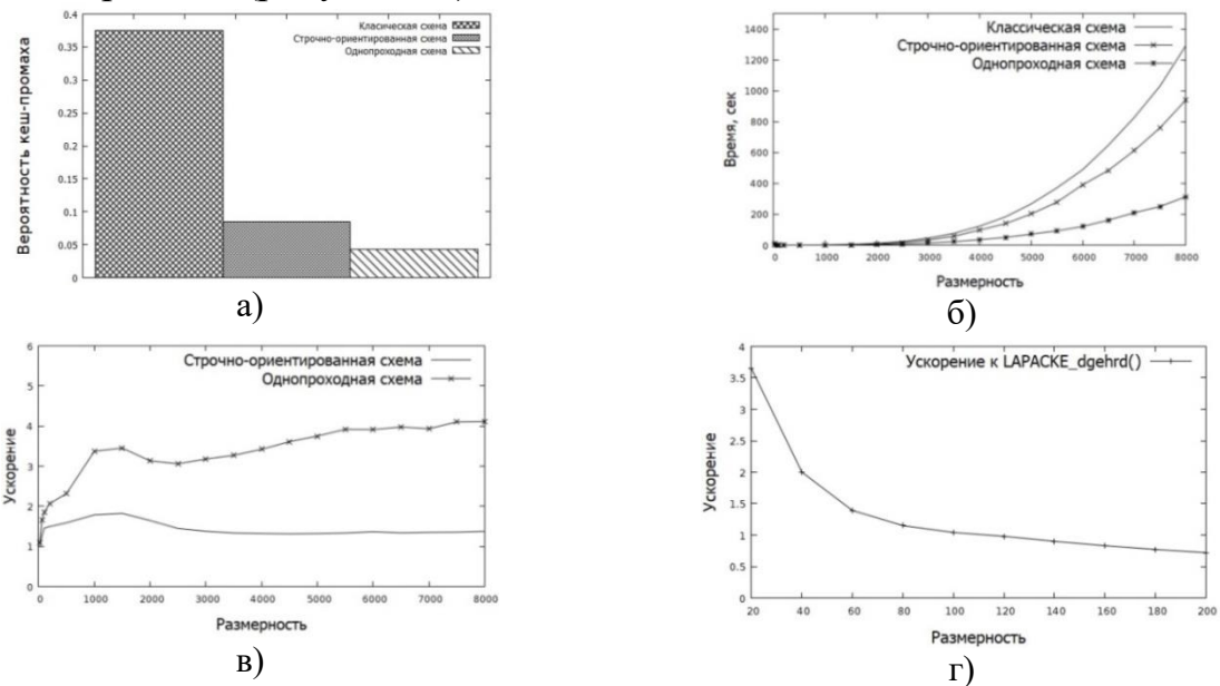
Рисунок 17 – Полученные метрики ПС: усредненное значение вероятности кеш-промаха (а), время работы (б), ускорение программы (в-г)
