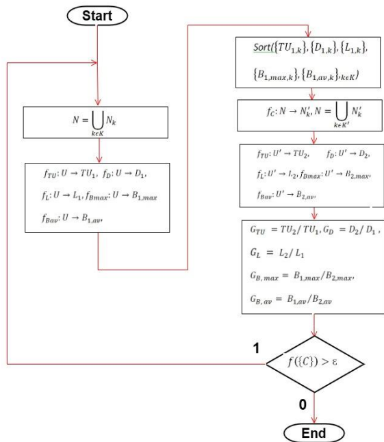
Рисунок 14 – Метод повышения эффективности использования GPU
