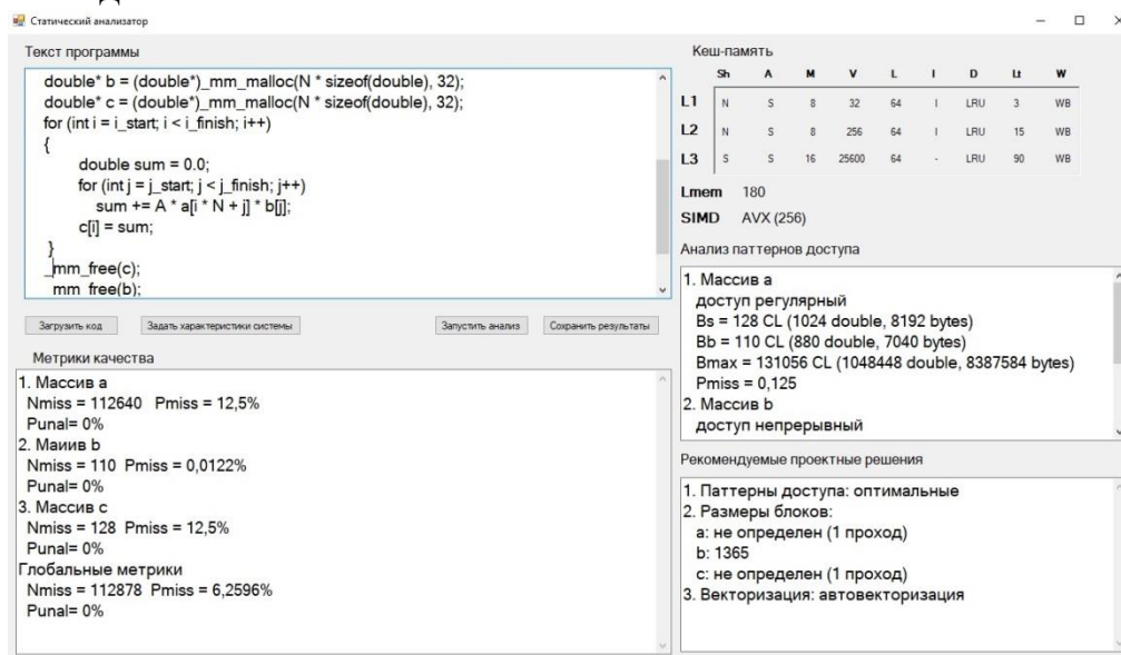
Рисунок 21 - Результаты формирования характеристик кода
