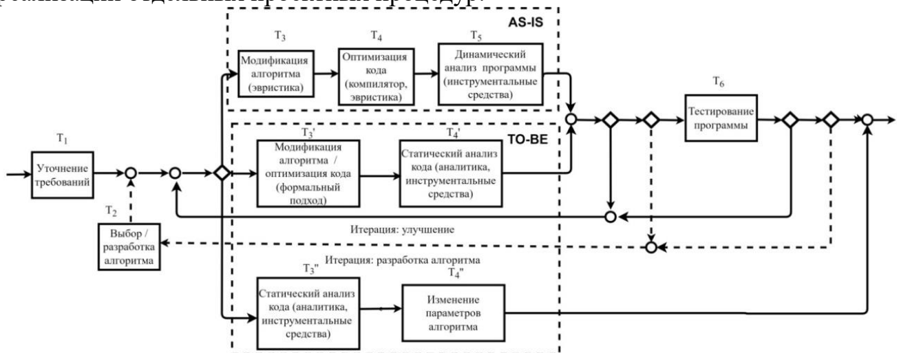
Рисунок 5 - Этап модификации ПС в соответствии с моделью улучшения показателей эффективности ПС
