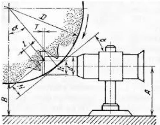
Рис. 1.5.2 – Схема экспериментальной установки для определения числа и разноразмерности зерен
