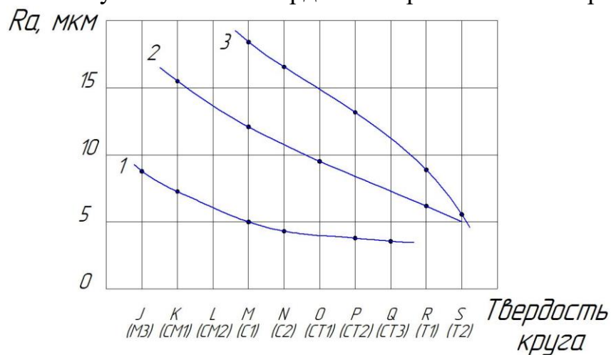
Рис. 1.2.1 – Зависимость высоты шероховатостей Rz от твердости кругов при разной их зернистости: 1- зернистость F90(16); 2 – зернистость F36(50); 3 – зернистость F24(80)
