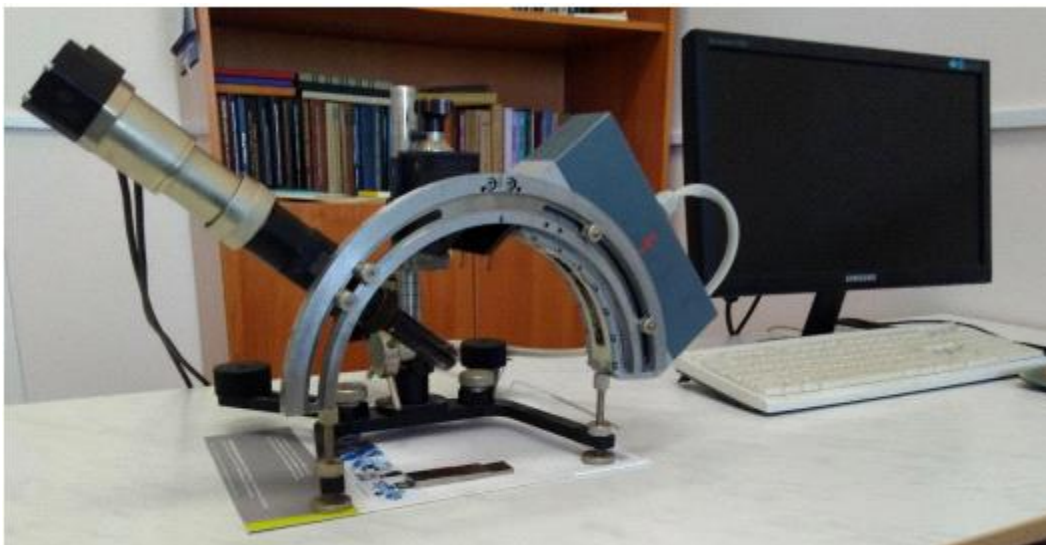
Рис. 4.1.5 – Рентгеновский измерительный комплекс для оценки неразрушающим методом остаточных напряжений "РИКОР-4"
