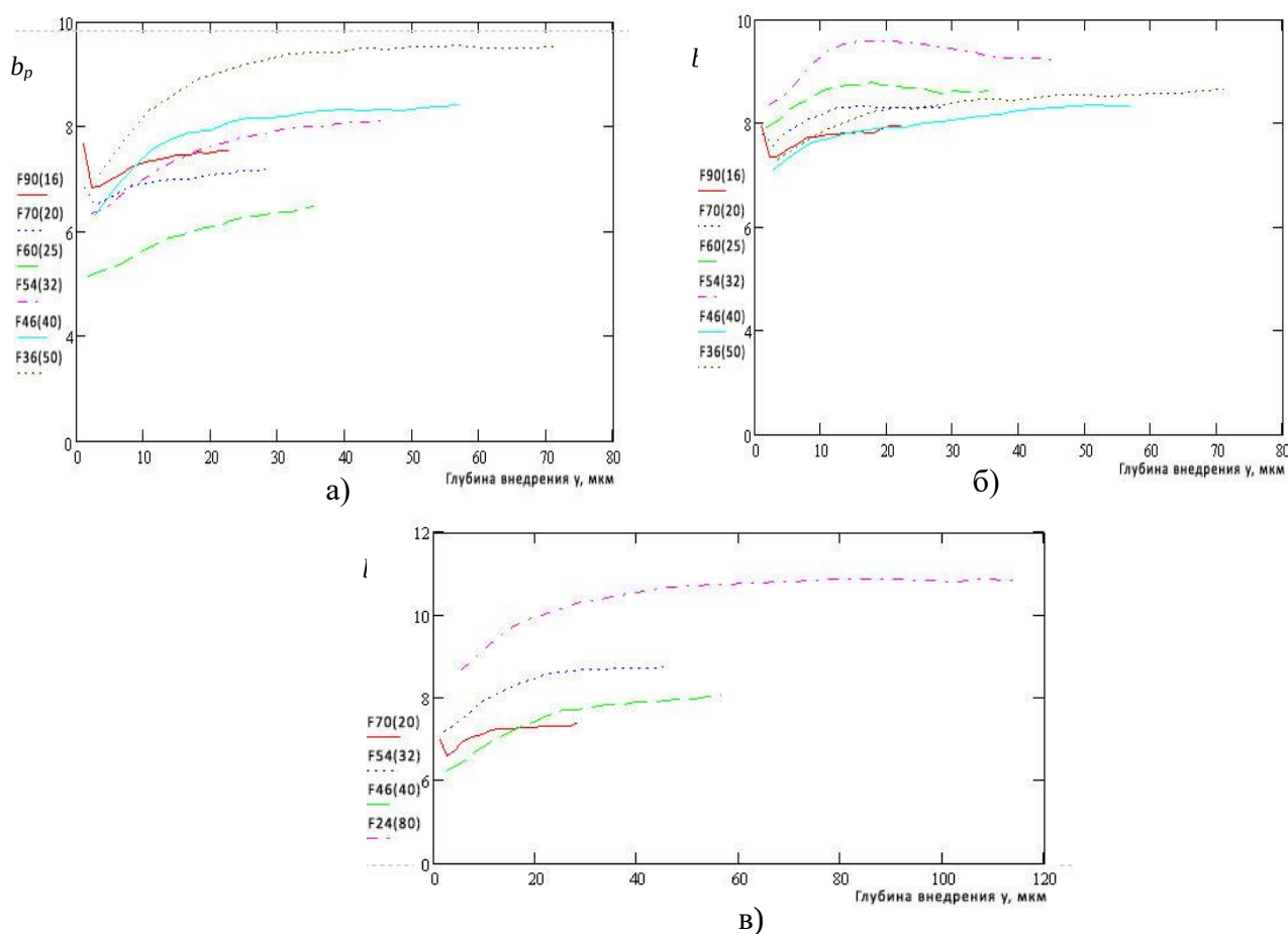
Рис. 3.1.16 – Значения средних параметров b_p для «деформирующих» кромок а) 53С; б) 63С; в) 92А
