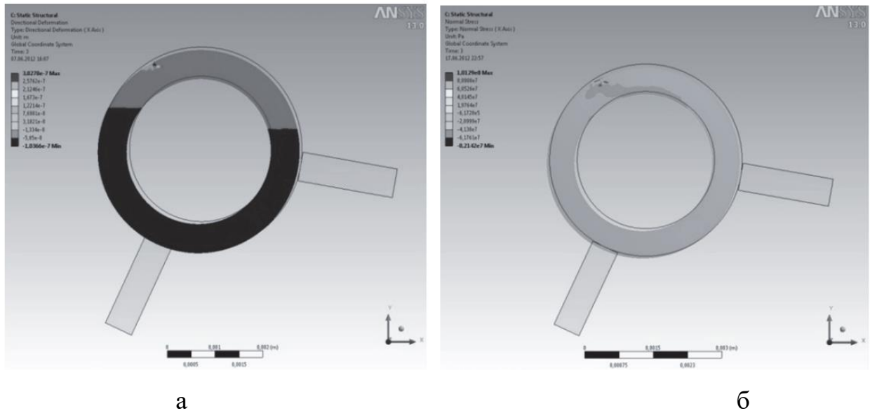
Рисунок 1.6.6 – Результат моделирования чернового режима шлифования внутреннего кольца подшипника в ANSYS Workbench при угле между опорой и горизонтальной осью кольца \alpha = 10^\circ : изолинии радиальных перемещений (а) и остаточных напряжений (б) [175]
