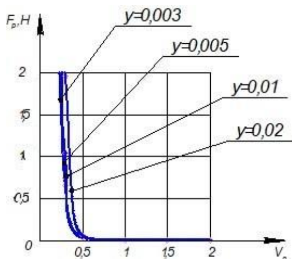
Рис.2.6.5 – График зависимости силы резания от формы а.з.
