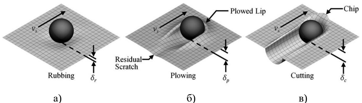
Рисунок 1.6.2 – Имитация удаления материала в программе LS-DYNA: притирание (а), вспашка (б) и резание (в) [172]
