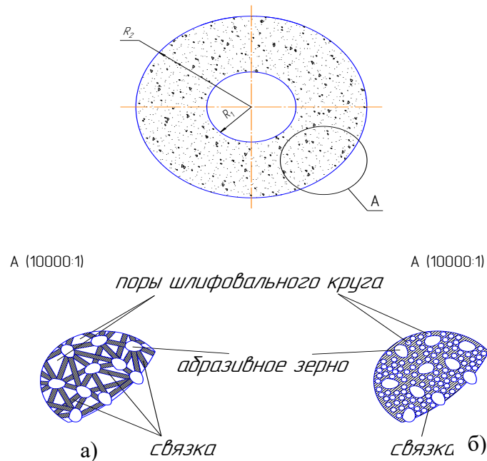
Рис.2.4.1 – Структура абразивного инструмента:
