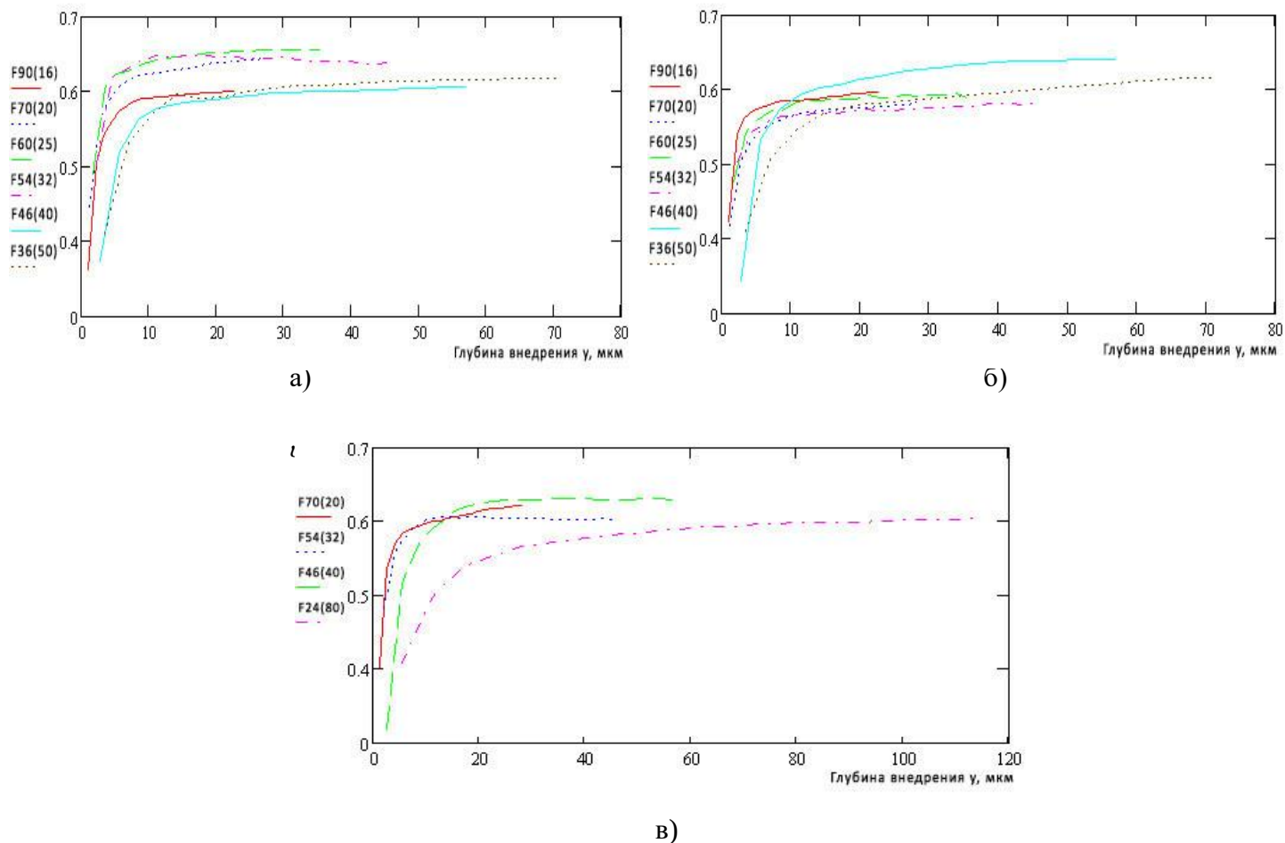
Рис. 3.1.19 – Значения средних параметров \nu_p для «режущих» кромок: а) 53С; б) 63С; в) 92А
