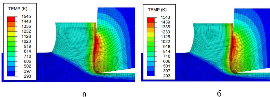
Рисунок 1.6.3 – Оценка распределения температуры в области контакта вершины режущей кромки с заготовкой из сплава AISI 4340 в программе Abaqus/Explicit: при \tau_p = 500 МПа (а) и при 700 МПа (б) [176]
