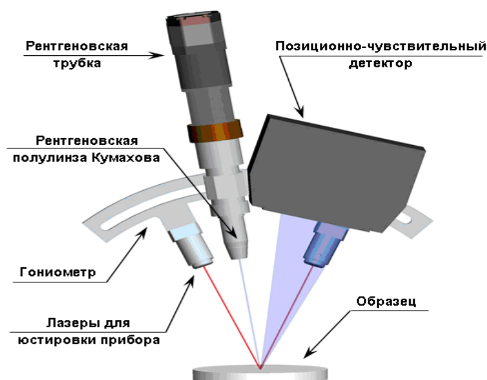
Рисунок 4.1.4 – Принципиальная схема устройства рентгеновского измерительного комплекса «РИКОР-4»
