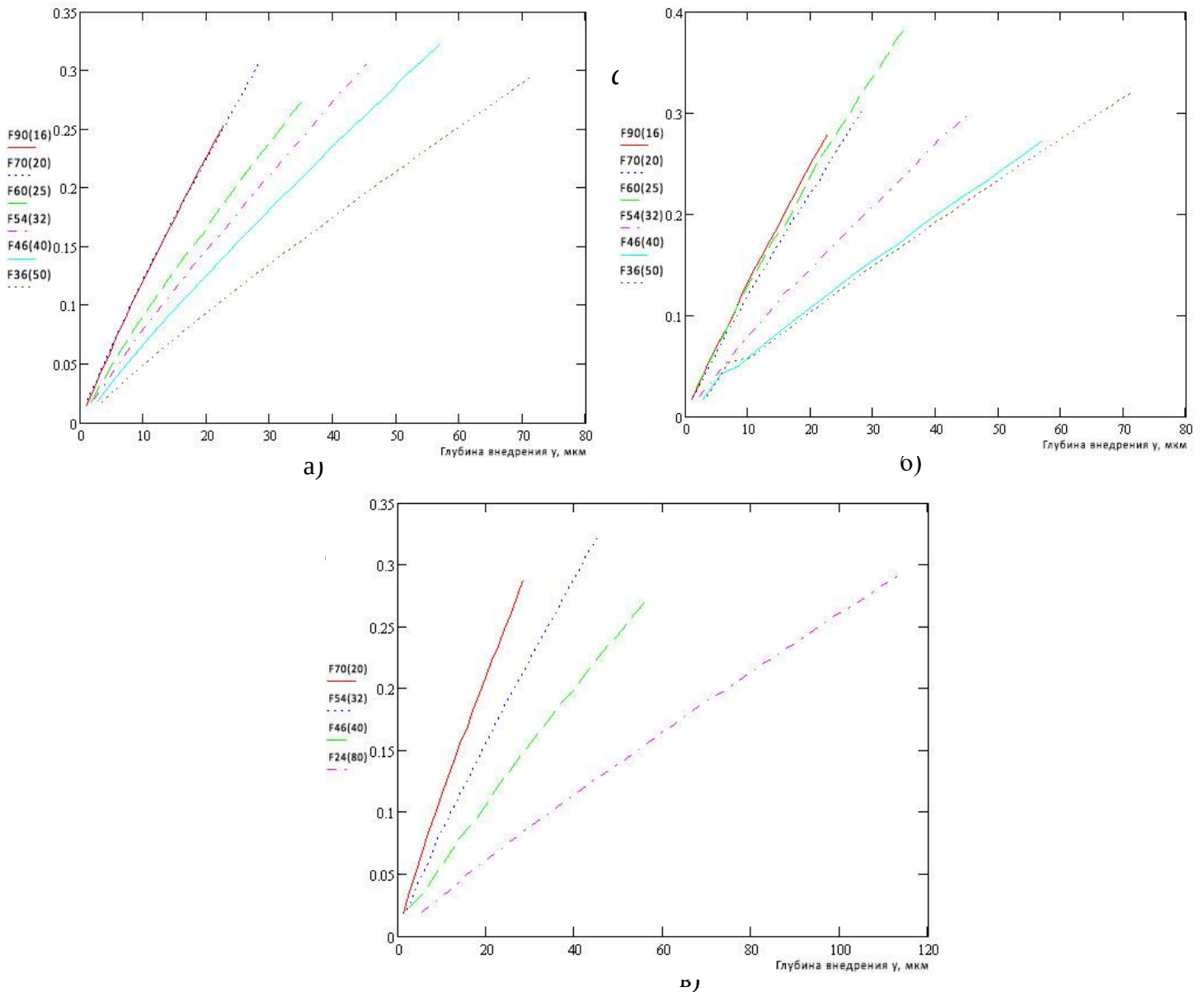
Рис. 3.1.23 – Средние значения критерия a_z/r
