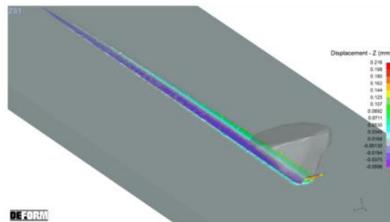
Рисунок 1.6.5 – Результат 3D-сканирования зерна абразива (геометрическая модель) (а), его конечно-элементное представление (б) и результат компьютерной симуляции процесса резания одиночным зерном в программе DEFORM 3D(в) [174]
