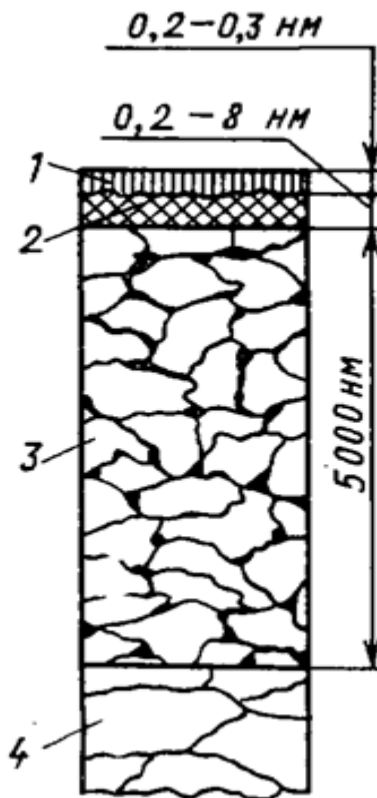
Рис. 1.3.1 – Схема строения поверхностного слоя металла [37]
