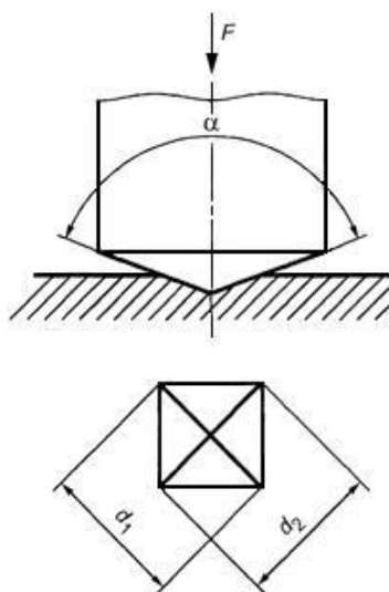
Рис. 4.1.6 – Схема приложения нагрузки
