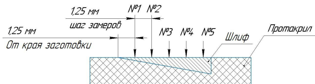
Рисунок 4.2.8 – Схема расположения точек, в которых производили измерение микротвердости
