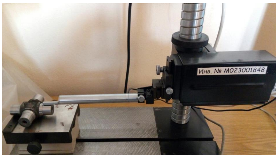
Рис. 4.1.1 – Профилометр модели 130
