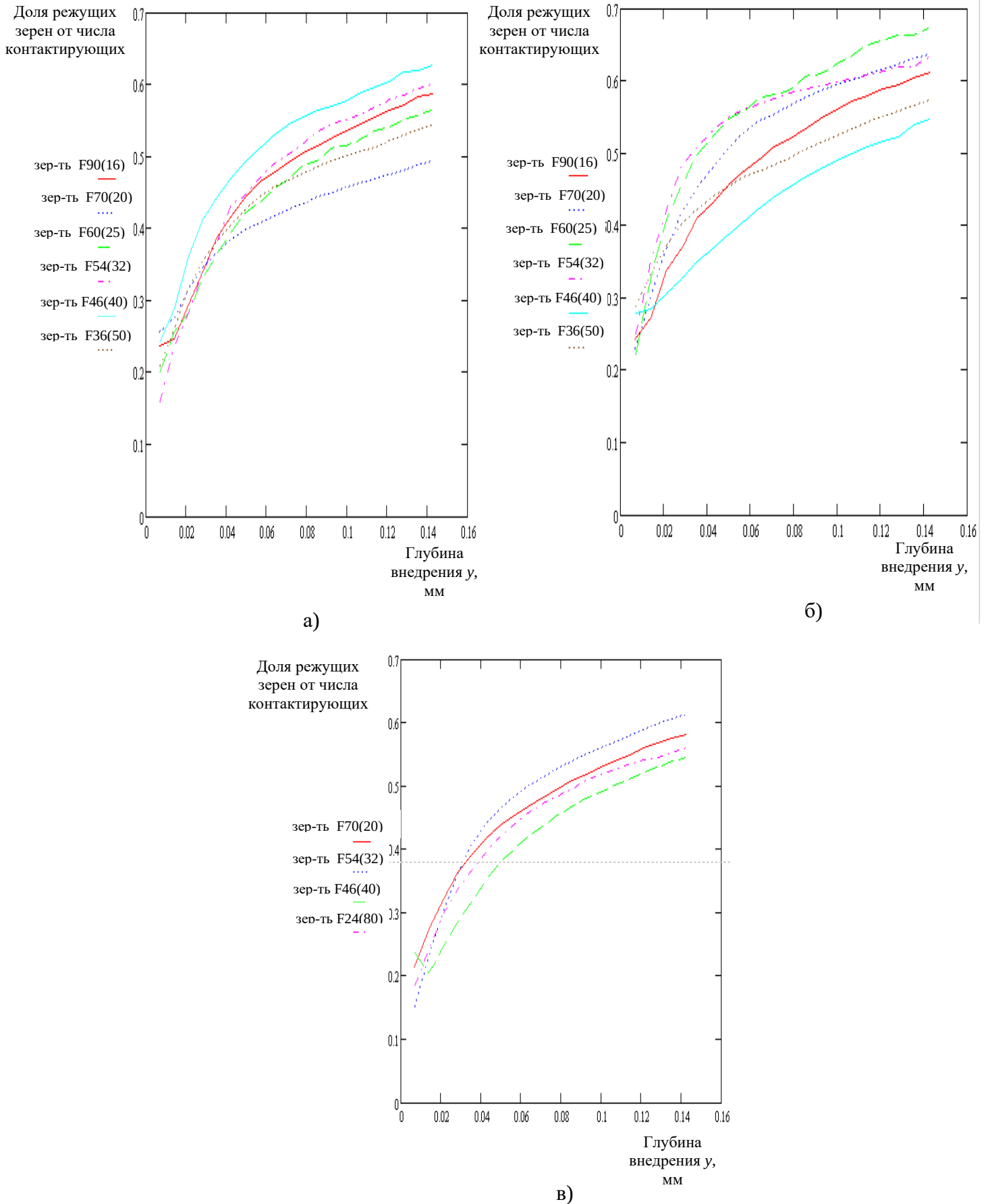
Рис.3.1.14 – Средние значения доли режущих зерен от числа контактирующих
