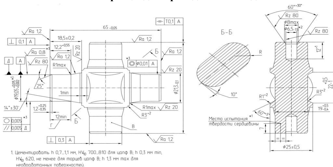
Рис. 4.2.9 – Чертеж заготовок для эксперимента
