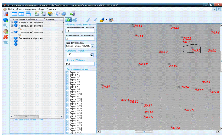
Рис. 3.3.2 – Подсчет зерен в программе ResFraction
