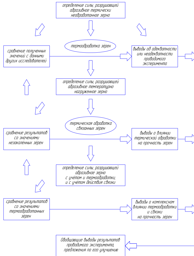
Рис.3.2.2 Алгоритм эксперимента
