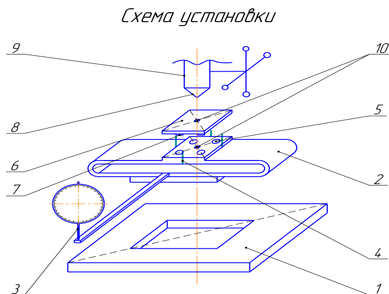
Рис.3.2.1. Схема приспособления, применяемого в эксперименте
