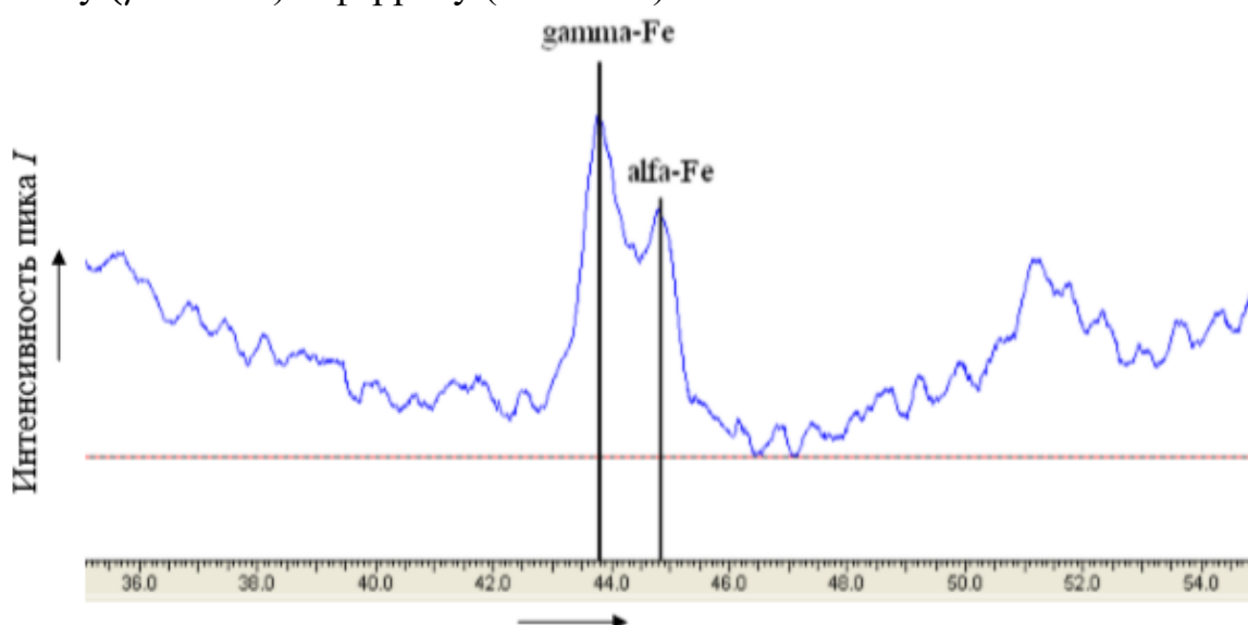
Рисунок 4.1.3 – Показания рентгеновского измерительного комплекса «Рикор-7»
