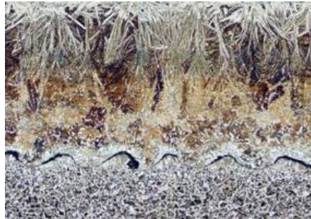
Интерметаллидные композиты
